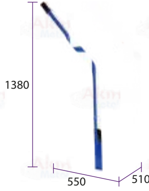
Varil Taşıma Arabası K-60.140
