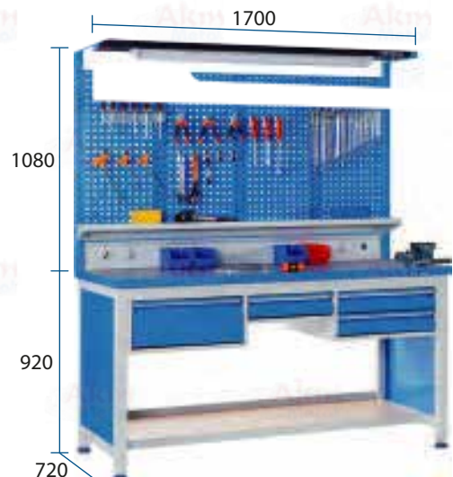
Profil Çalışma Tezgahı A-15.862
