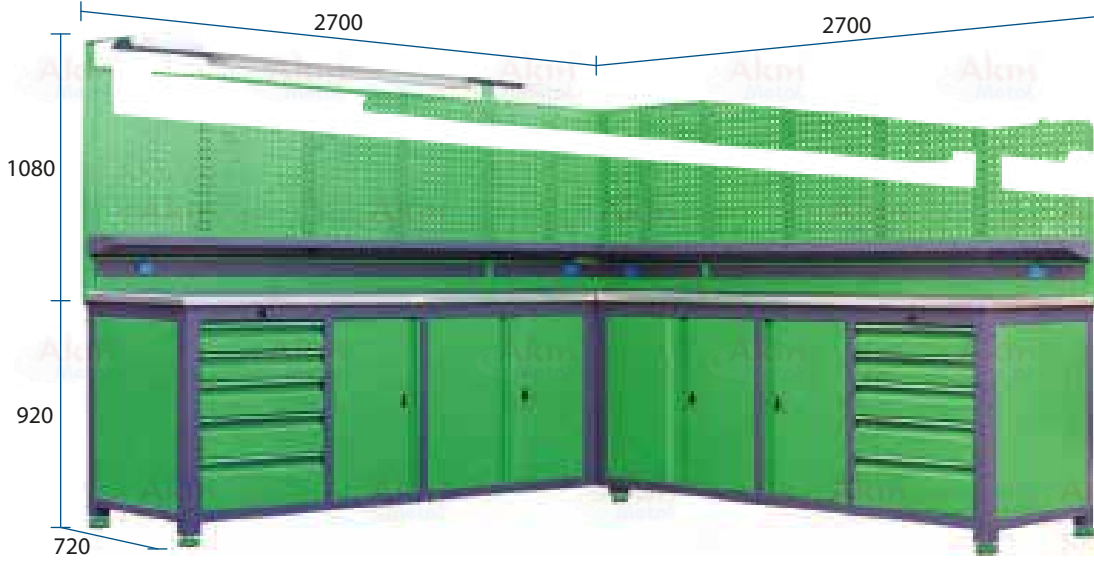
Profil Çalışma Tezgahı A-15.754
