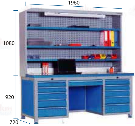
Profil Çalışma Tezgahı A-15.858
