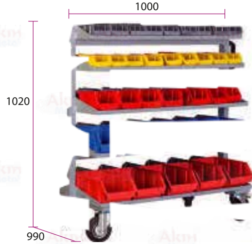
Avadanlık Standı P-90.128
