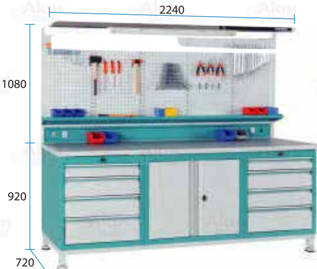
Modüler Çalışma Tezgahı B-20.130
