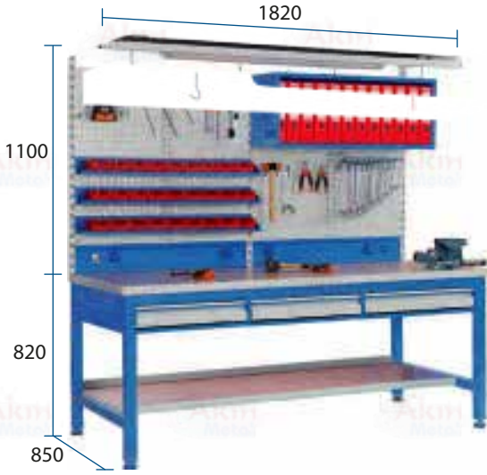
Profil Çalışma Tezgahı A-15.868
