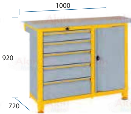
Profil Çalışma Tezgahı A-15.226
