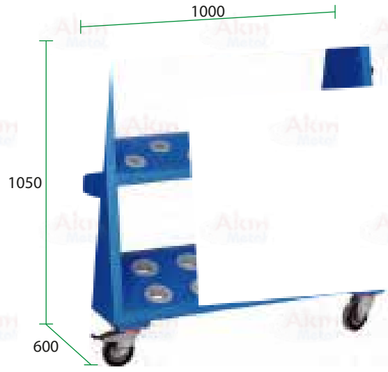
Mors Tutucu Arabası E52
