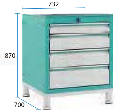
Modüler Çalışma Tezgahı B-21.114
