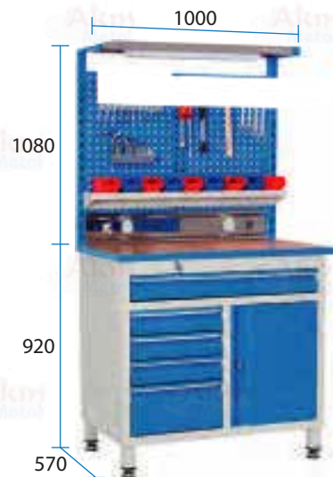
Modüler Çalışma Tezgahı B-20.122
