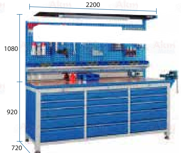
Profil Çalışma Tezgahı A-10.116
