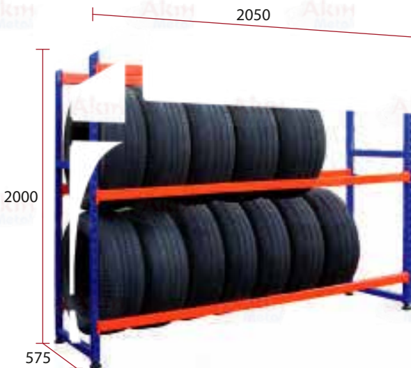
Lastik İstifleme Rafı L-65.116
