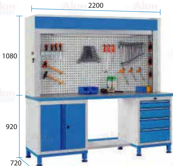
Modüler Çalışma Tezgahı B-22.102
