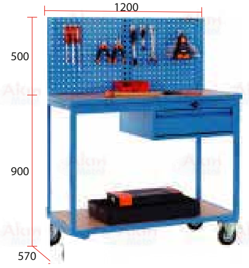
Takım Arabası D-30.314
