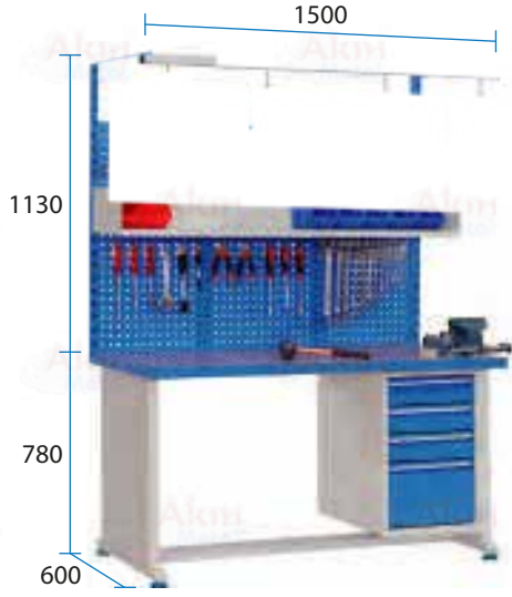
Modüler Çalışma Tezgahı B-20.200
