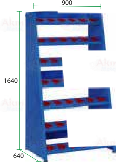
Mors Tutucu Raflı R5 E-30
