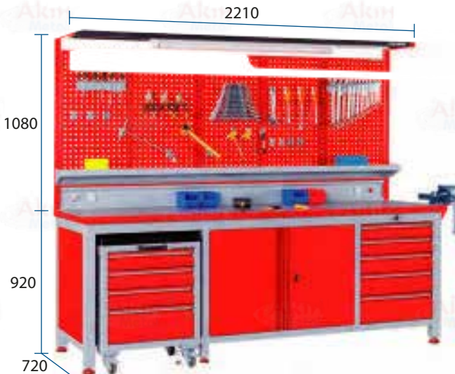
Profil Çalışma Tezgahı A-15.602
