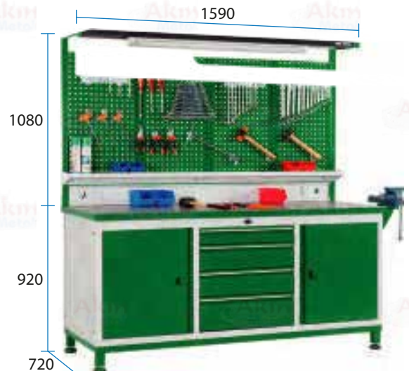
Modüler Çalışma Tezgahı B-20.108
