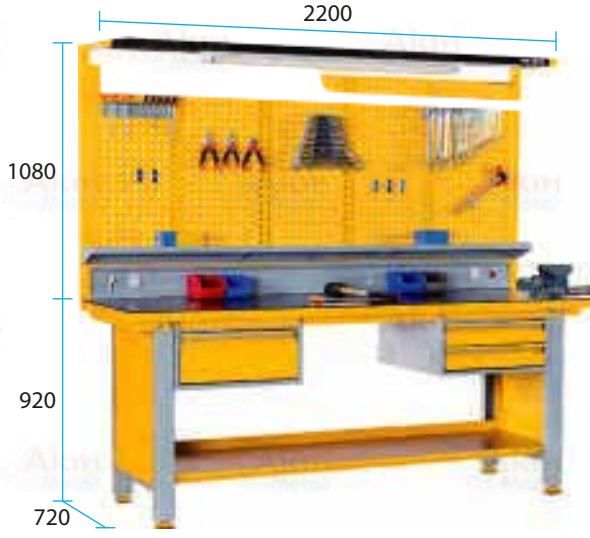
Demonte Çalışma Tezgahı C-25.112
