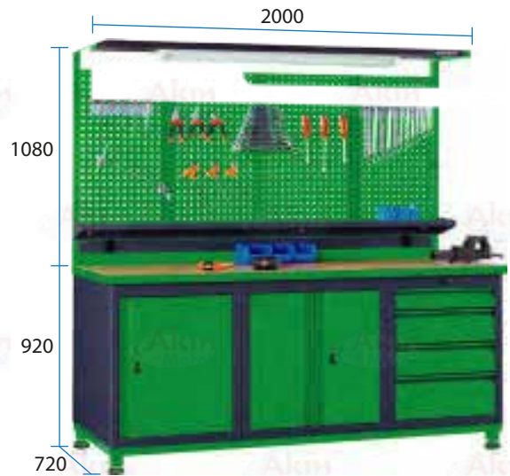
Modüler Çalışma Tezgahı B-20.156
