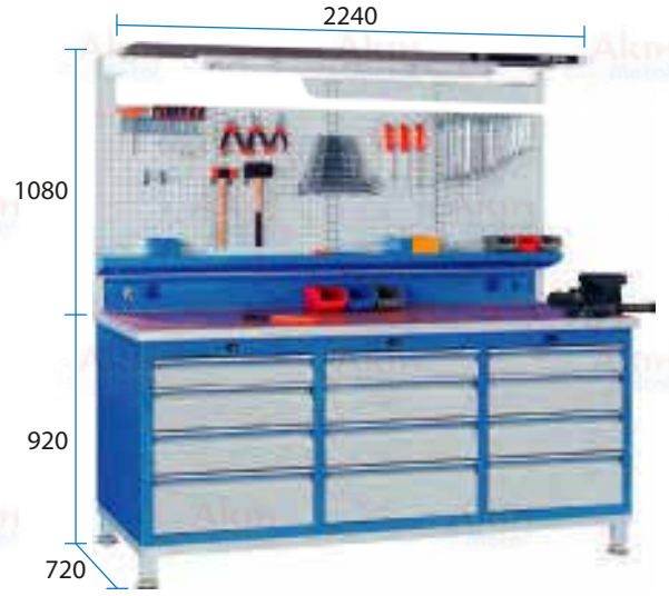
Modüler Çalışma Tezgahı B-20.116
