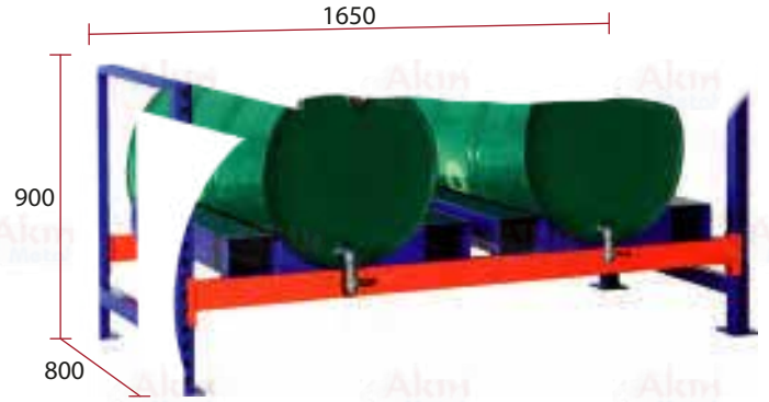
Konsol Kollu Stok Rafı L-65.118
