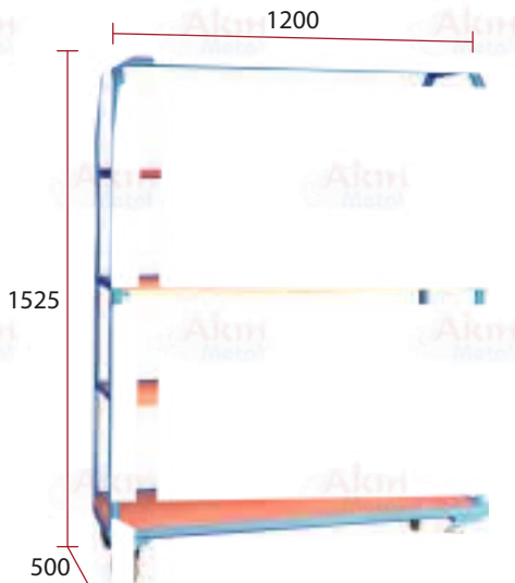
Malzeme Rafı L-65.202
