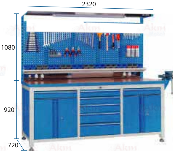
Profil Çalışma Tezgahı A-15.514
