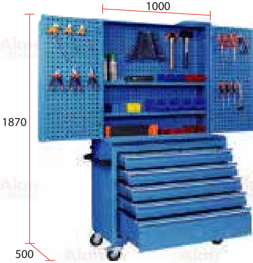
Takım Arabası D-30.502
