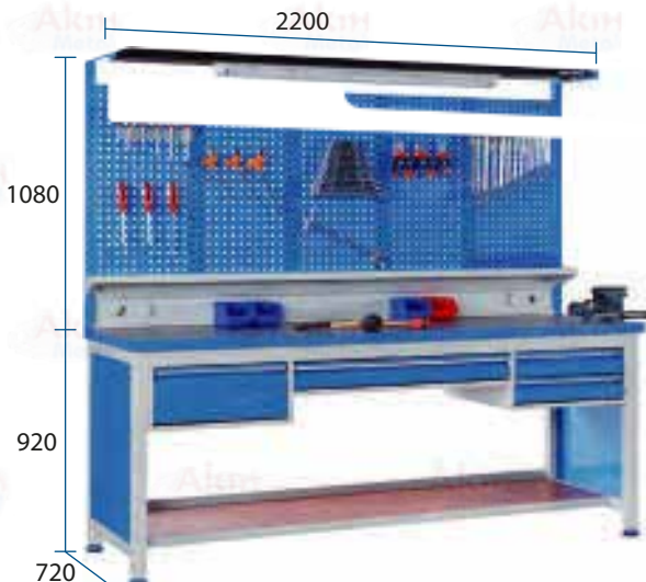
Profil Çalışma Tezgahı A-15.860
