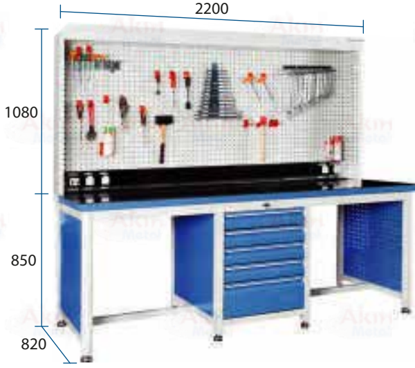
Profil Çalışma Tezgahı A-15.856
