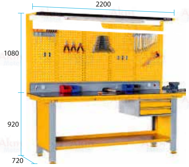
Demonte Çalışma Tezgahı C-25.302
