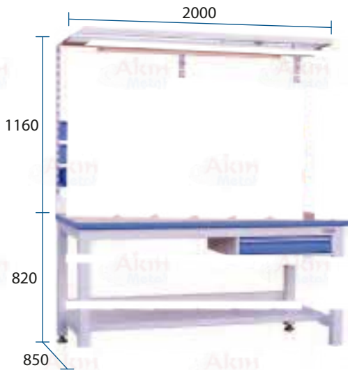
Profil Çalışma Tezgahı A-17.102
