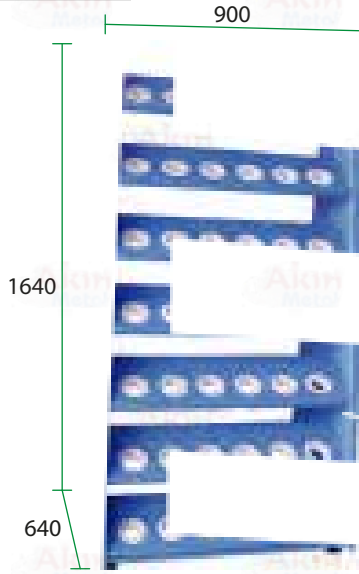
Mors Tutucu Raflı R5 E-32
