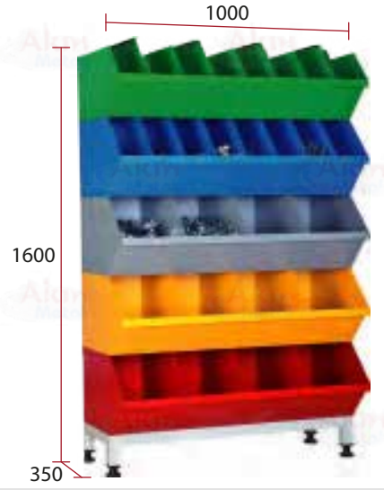
Fittings Stok Rafı L-65.148
