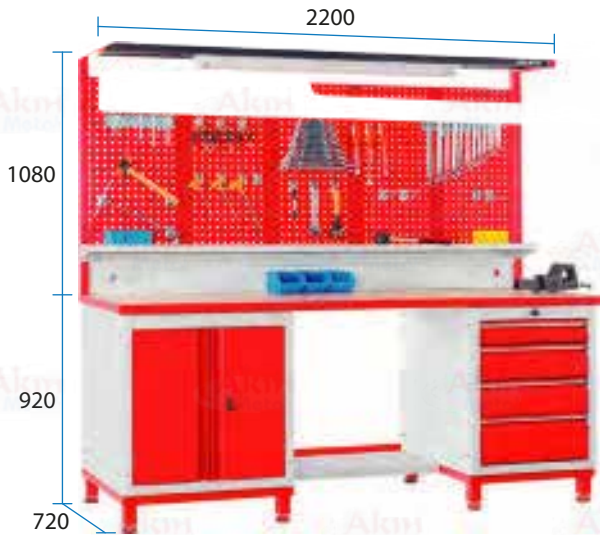
Modüler Çalışma Tezgahı B-20.120
