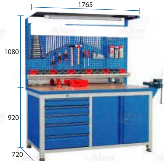
Profil Çalışma Tezgahı A-10.116
