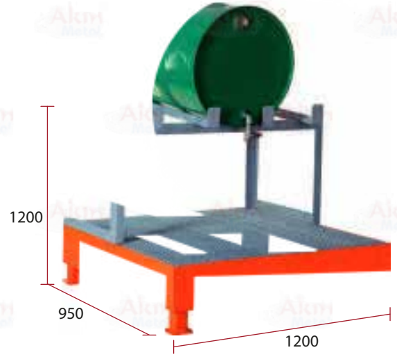
Varil Sehpaı L-65.115
