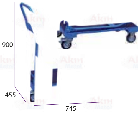
Paket Taşıma Arabası K-60.118
